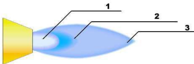
Рис.1 Строение сварочного пламени.
