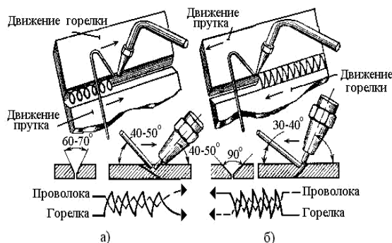
Рис.1 Способы газовой сварки: а- левый; б – правый.
