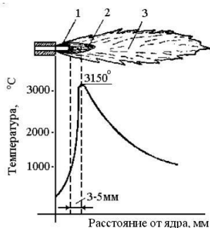
Рис. 2. Строение сварочного ацетилено-кислородного пламени:
