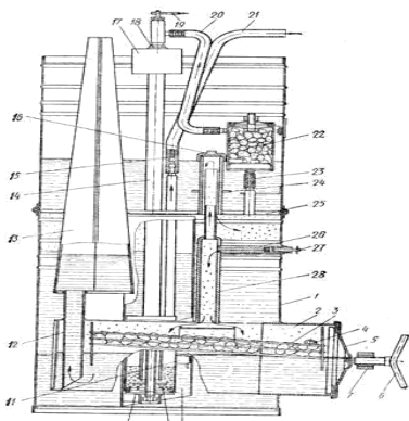
Рис.1 Ацетиленовый генератор АНВ-1,25
